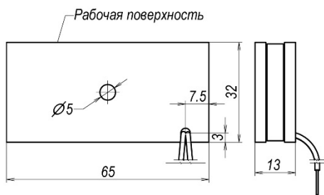
Рисунок 1 - Корпус
