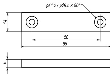
Рисунок 2 – Якорь
