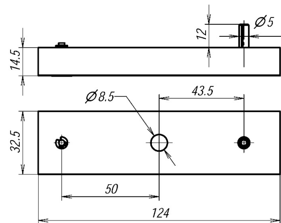
Рисунок 7 - Якорь
