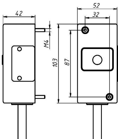
Рисунок 1 - Габаритно-установочные размеры счетчика AL-RD-05 (вариант К)
